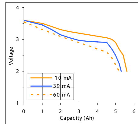
150°C discharge
