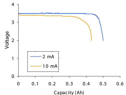
150°C discharge
